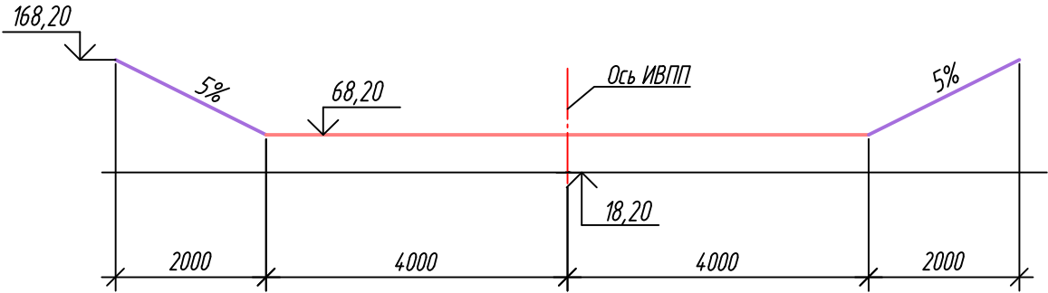
Разрез 2-2 М 1:100 000 – по горизонтали М 1:10 000 – по вертикали
