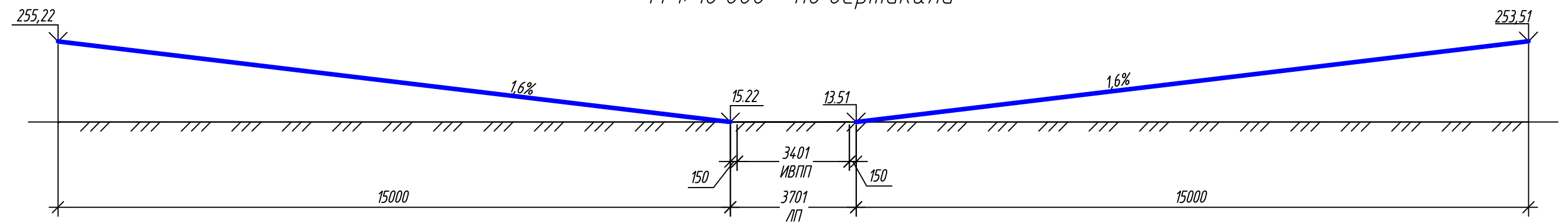
Разрез 1-1 М 1:100 000 – по горизонтали М 1: 10 000 – по вертикали
